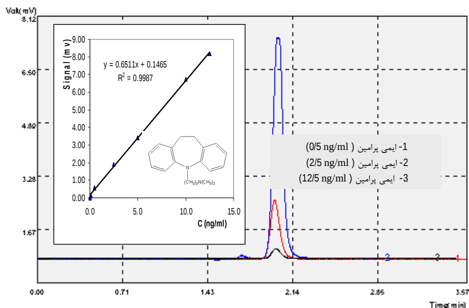
شکل 1. کروماتوگرام و منحنی کالیبراسیون ایمی پرامین مربوط به تعیین مقدار ماده مؤثره و میزان یکنواختی ایمی پرامین در قرص های 10 و 50 میلی گرمی (شرایط دستگاهی شامل ستون: PRP-1 (4/1 × 150 mm ، 10 μm) در دمای +40°C ، فاز متحرک: استونیتریل: محلول بافر فسفات (62:38 در pH=4/0) با سرعت جریان 1/5 ml/min، طول موج تهییج: 250 نانومتر و طول موج نشر فلورسانس: 360 نانومتر)
